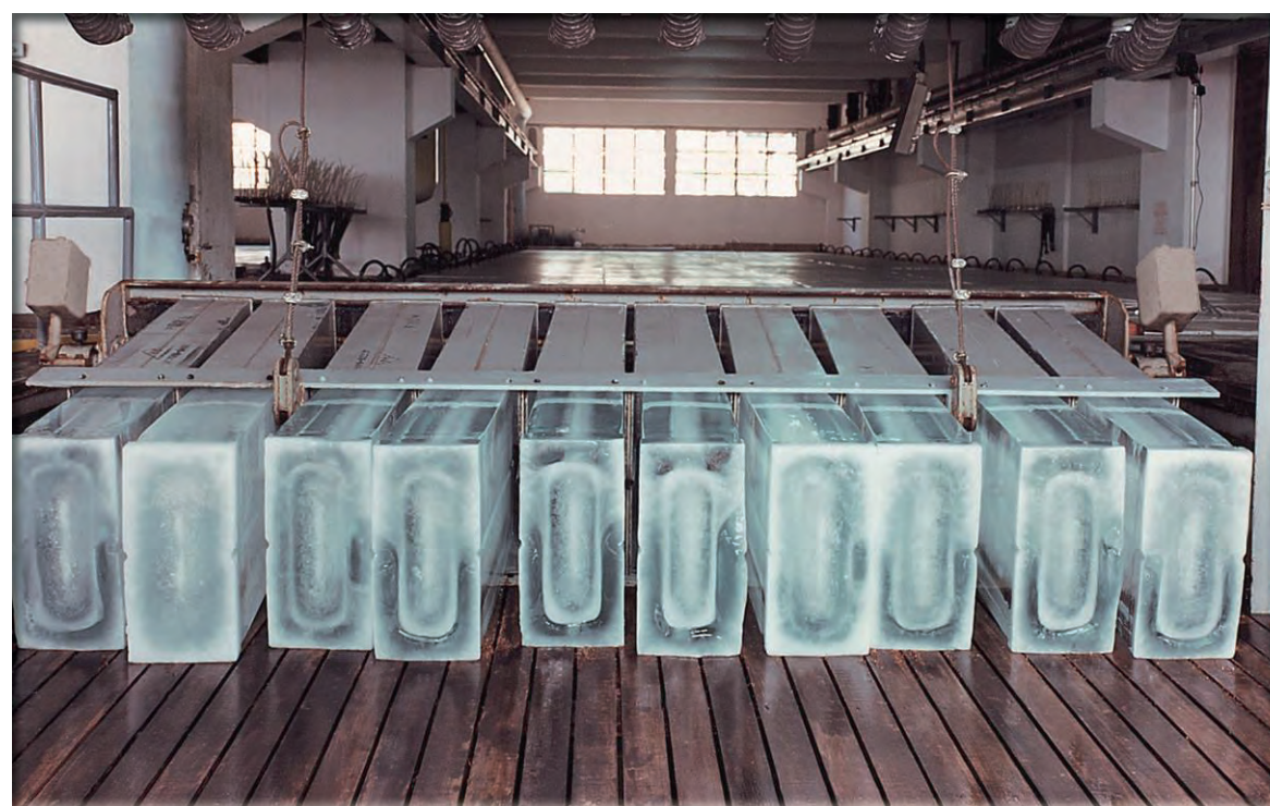
Fabrica de Bloques de Hielo
